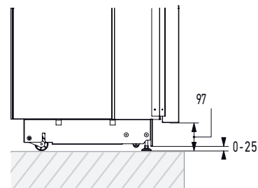
PLINTH SIZE
