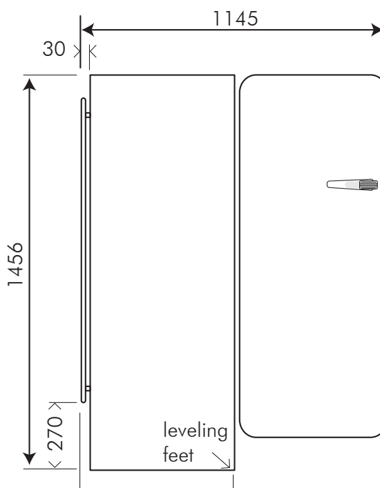
SIDE ELEVATION — door open
