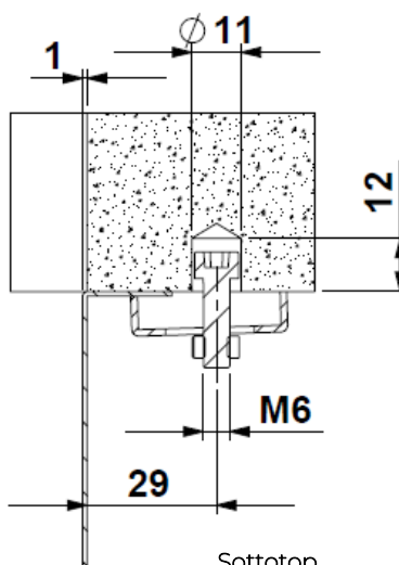
Sottotop Dettaglio di fissaggio Under mount Fastening detail
