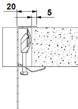
Sopratop Dettaglio di fissaggio Top mount Fastening detail
