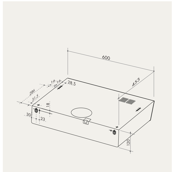
ASO601X | ASO901X ASO620X | ASO920X
